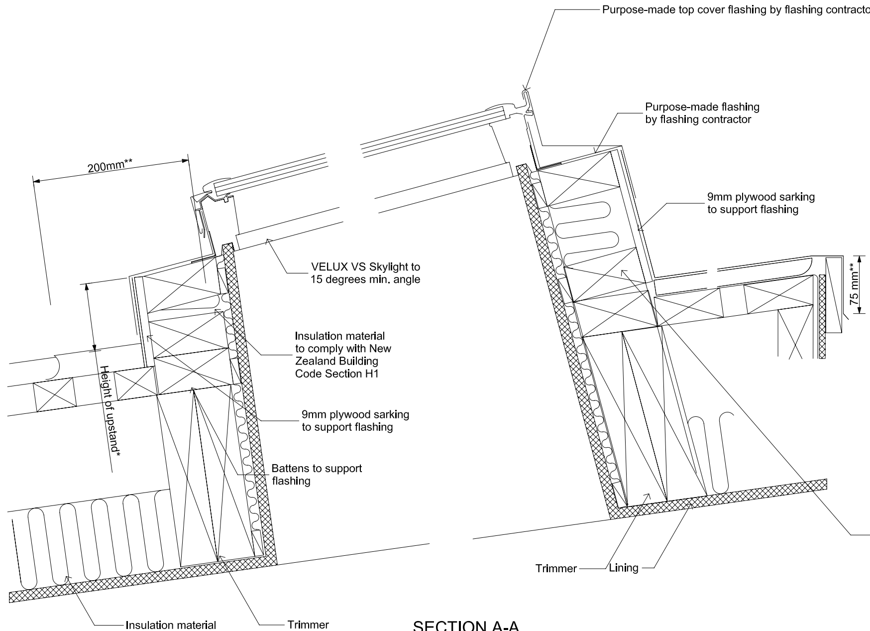
SECTION A-A
